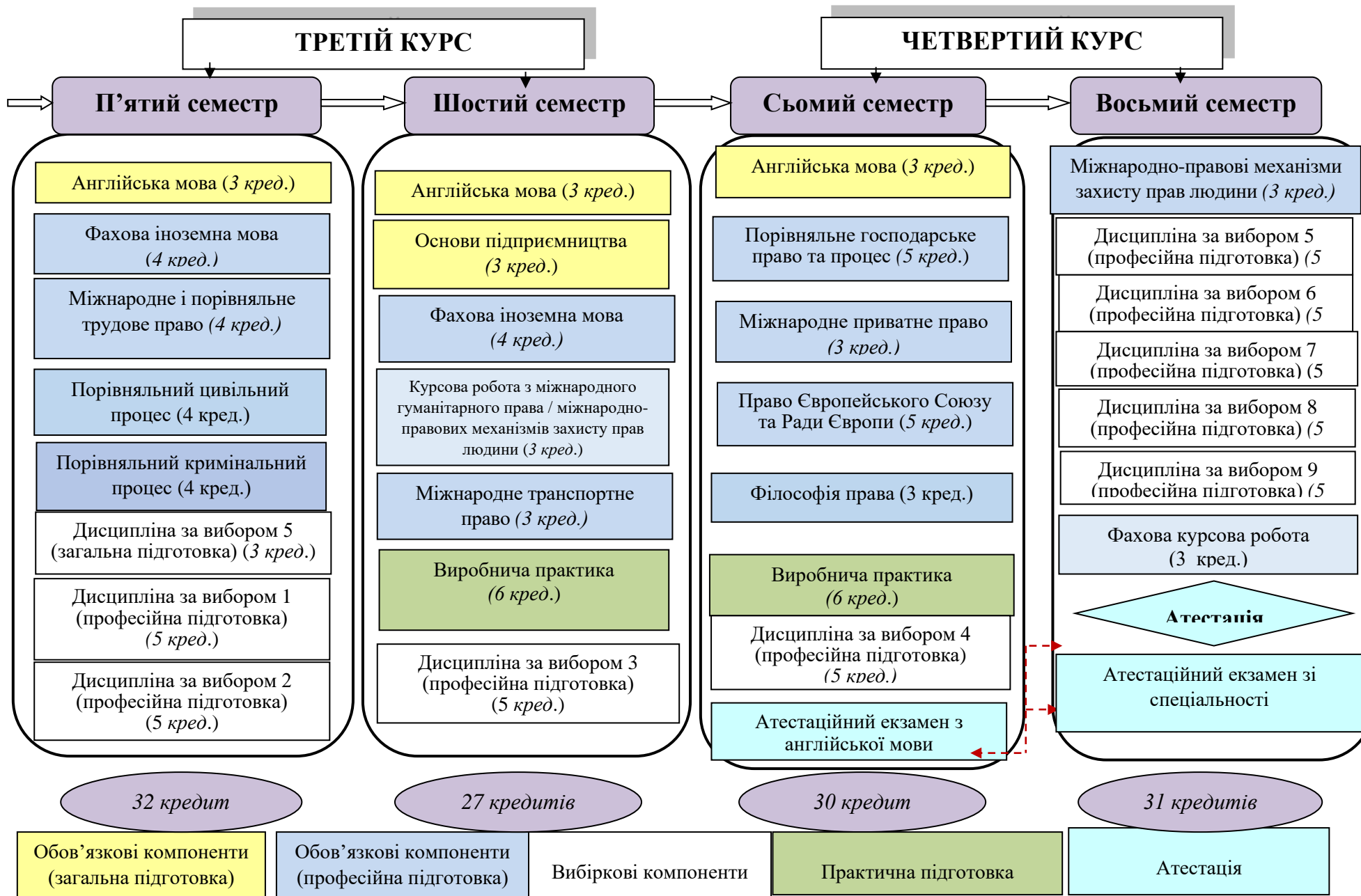
Рис. 1 Структурно-логічна схема
